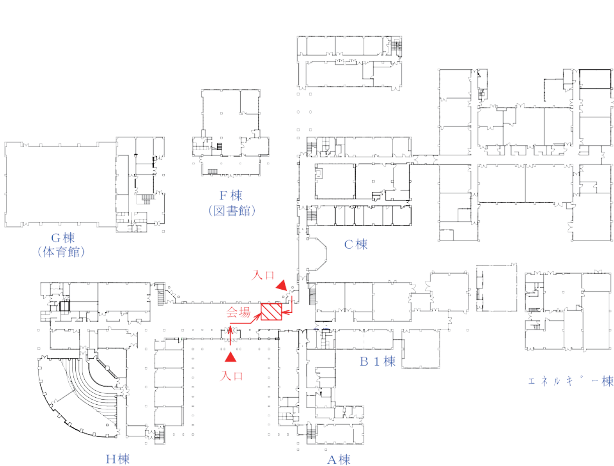
高岡キャンパス 1 階平面図
